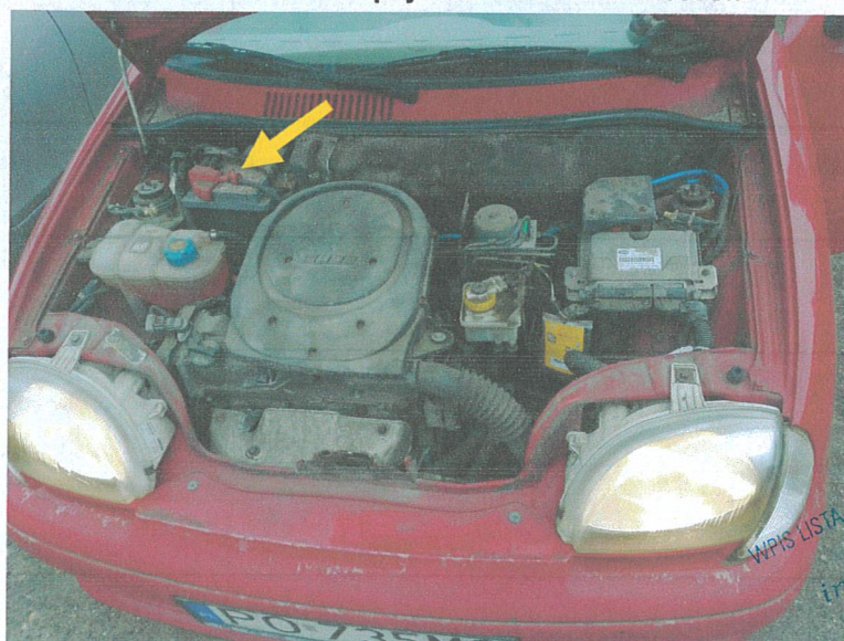
Fot. nr 6. Badania pojazdu – zakres uszkodzeń
